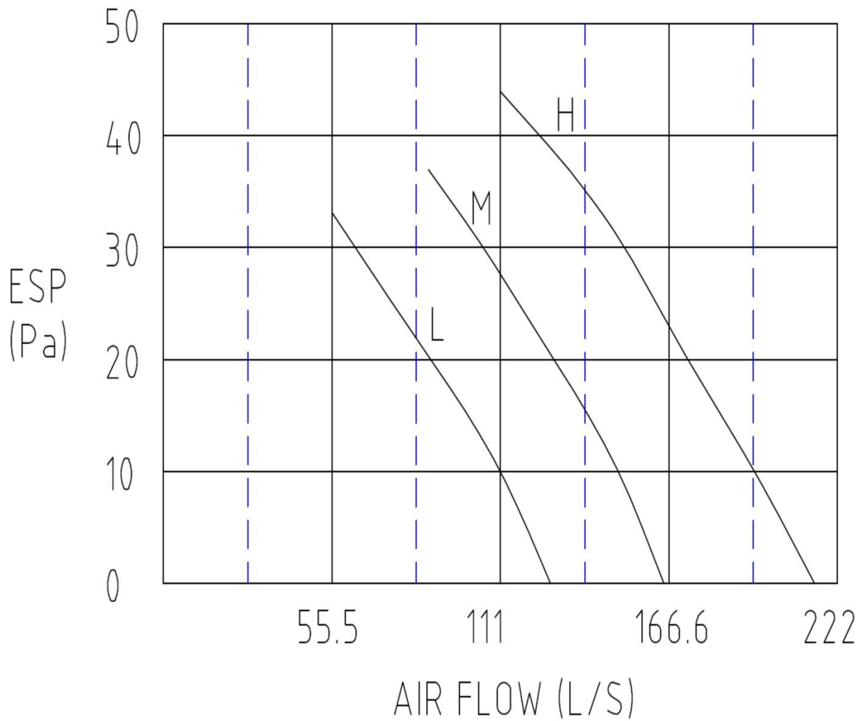
FAN CURVE
