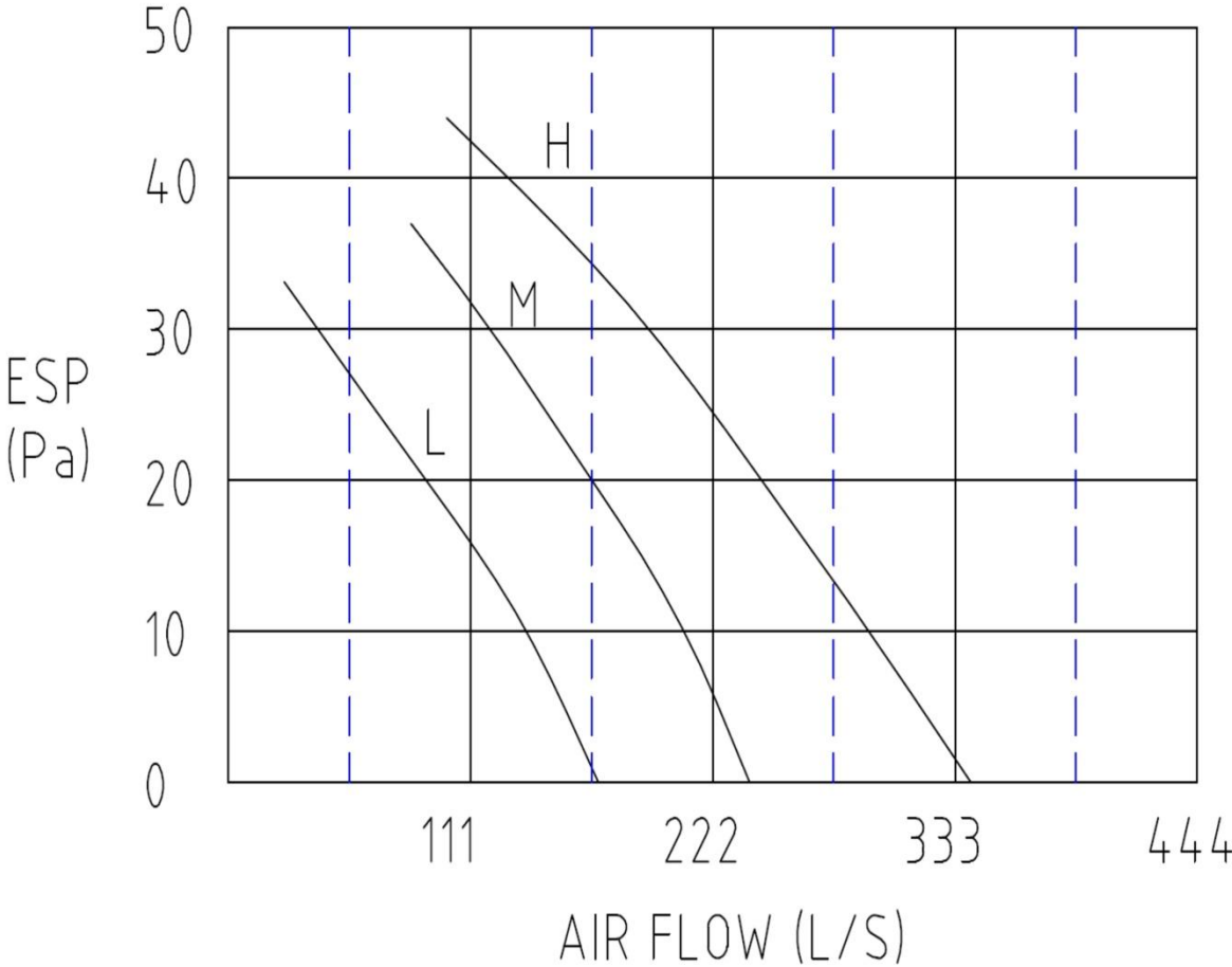
FAN CURVE
