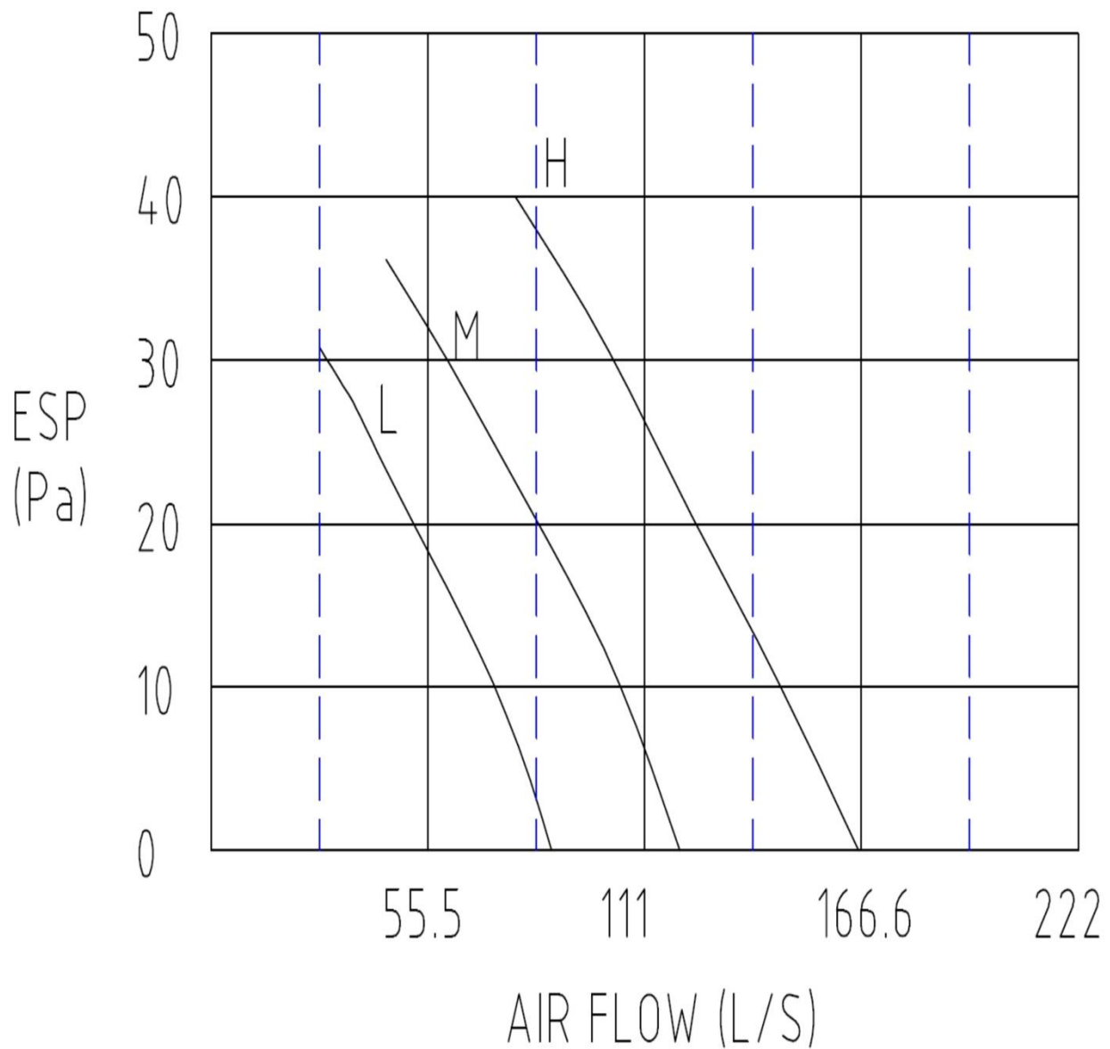
FAN CURVE
