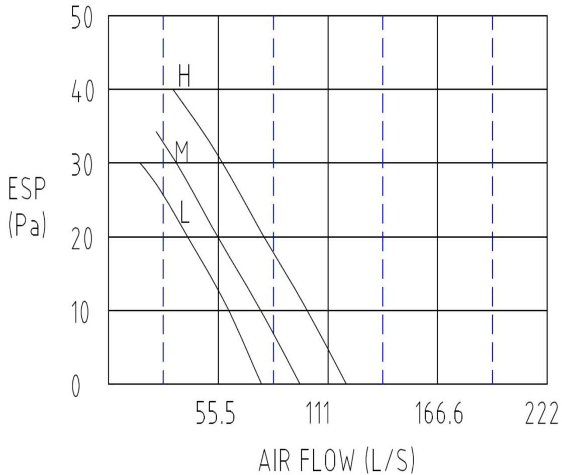
FAN CURVE
