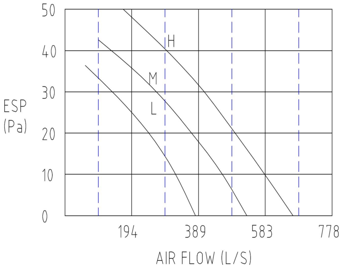
FAN CURVE
